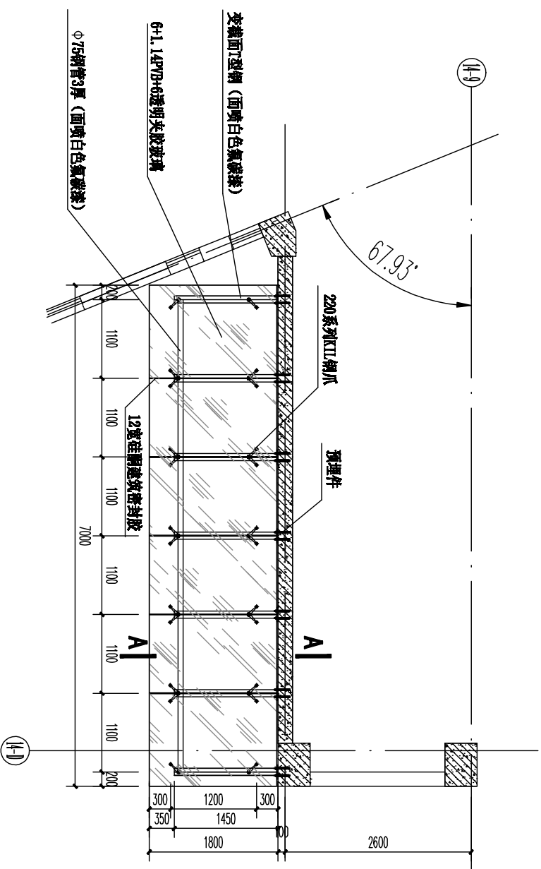
雨篷(A)平面布置图
