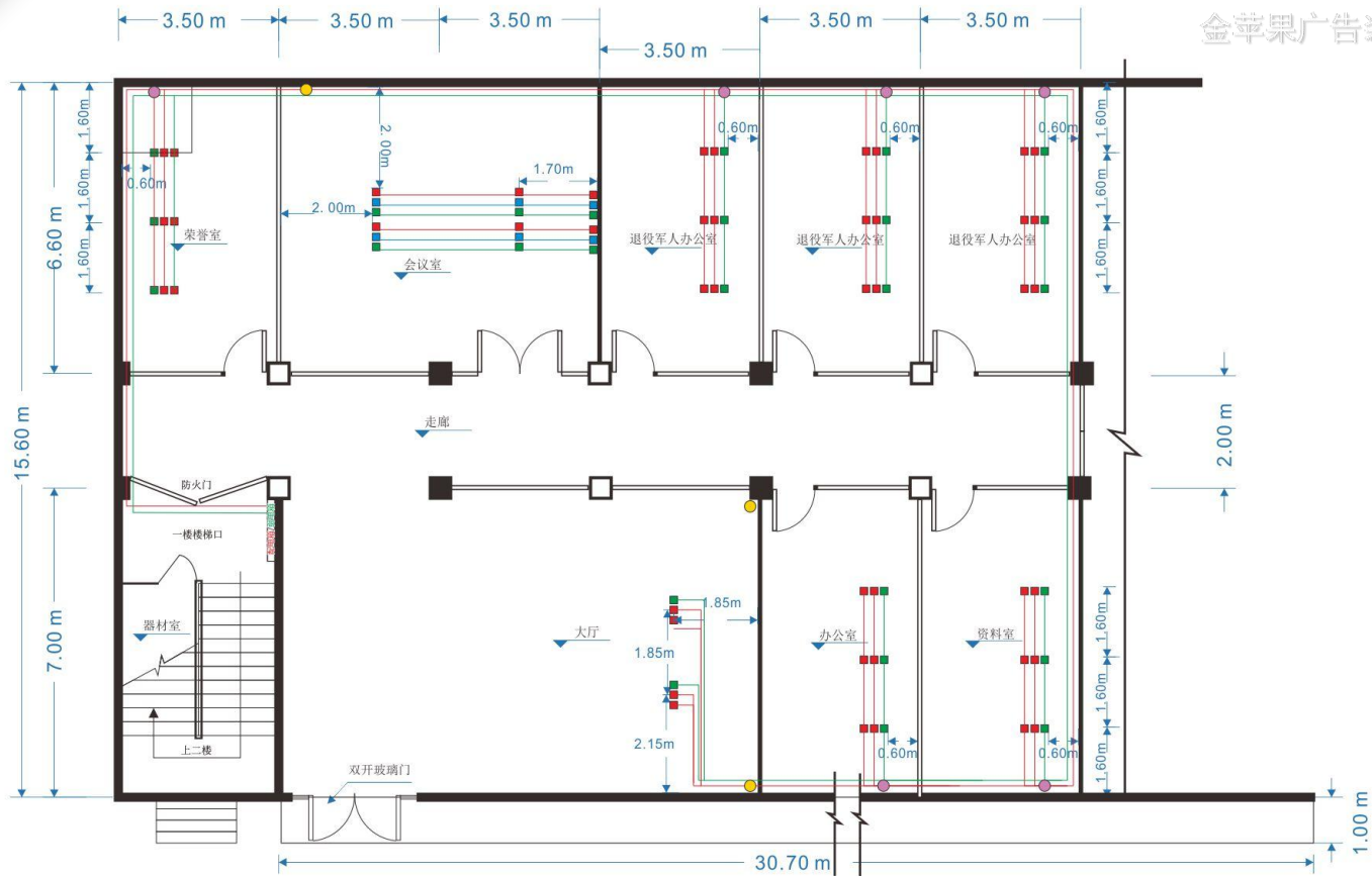
地插并联线路走向走势图
