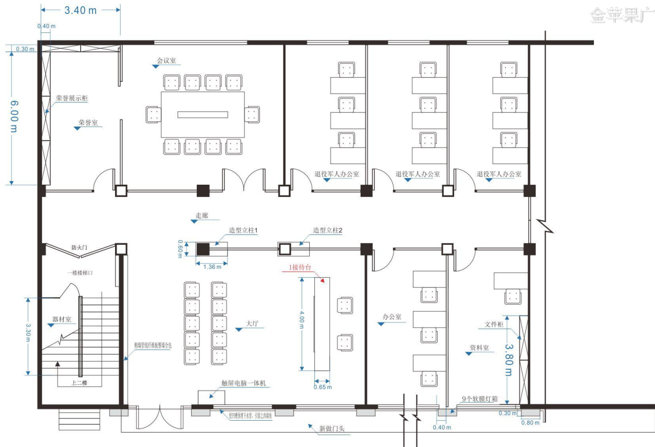
改造后布置平面图
