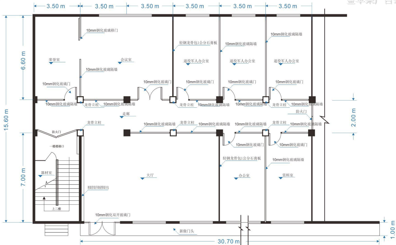
改造后平面尺寸图
