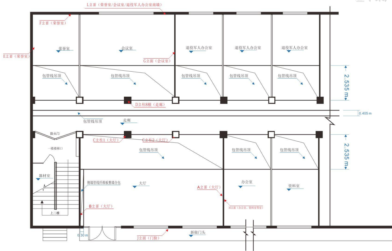
改造后顶部尺寸图
