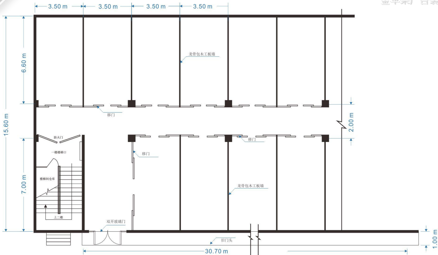
原平面尺寸图
