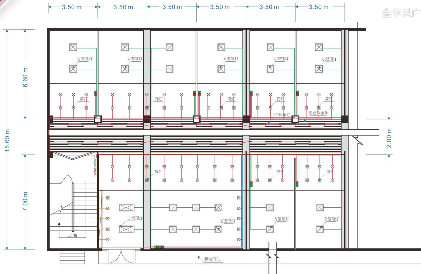
顶部灯光并联线路走势图
