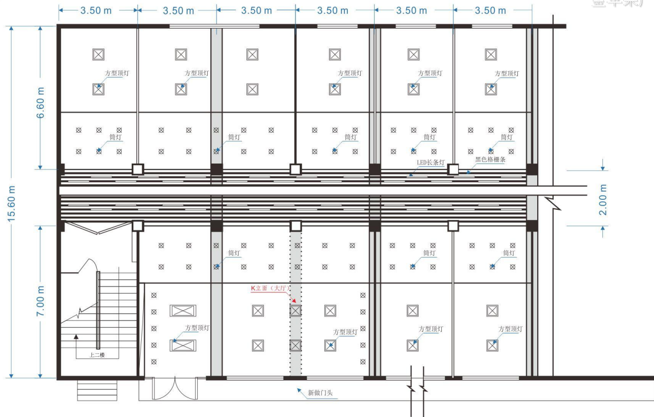
改造后顶部灯光布置图
